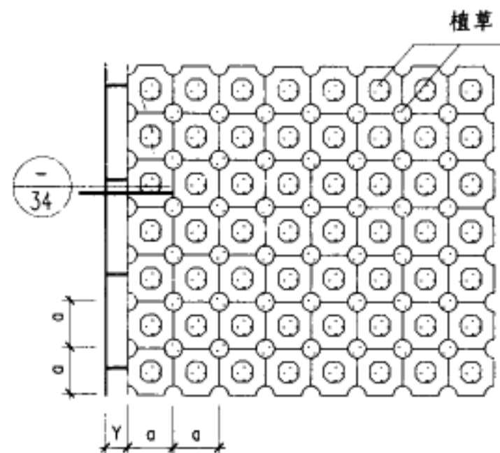
③ 型嵌草砖
