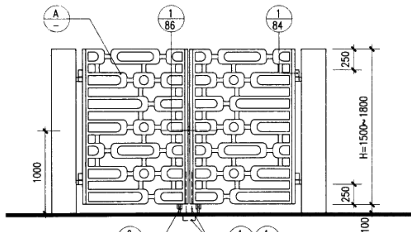
立面
