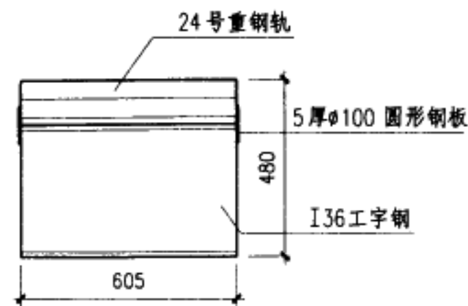
侧立面图
