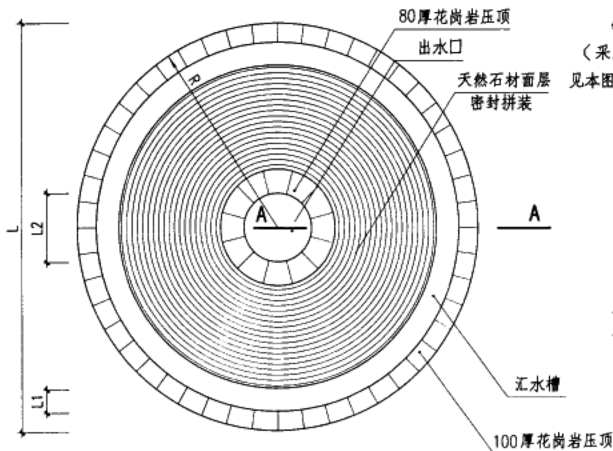
2a 2b 2c 2d 平面
