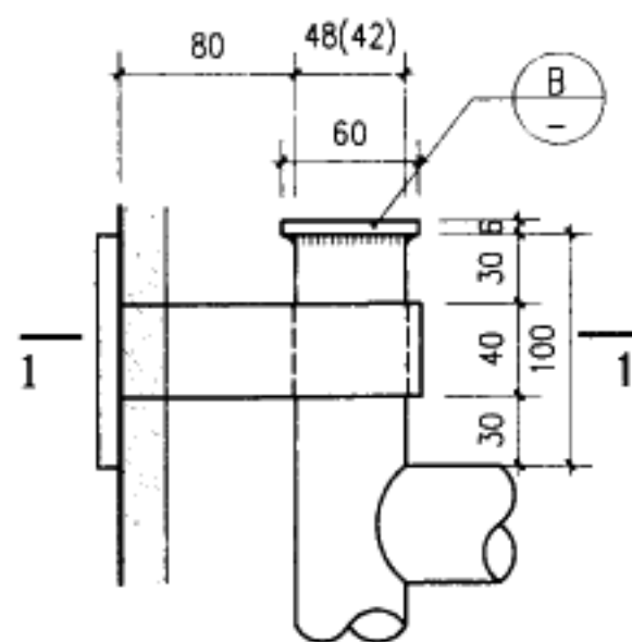
上轴立面
