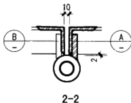
用于角钢边框门
