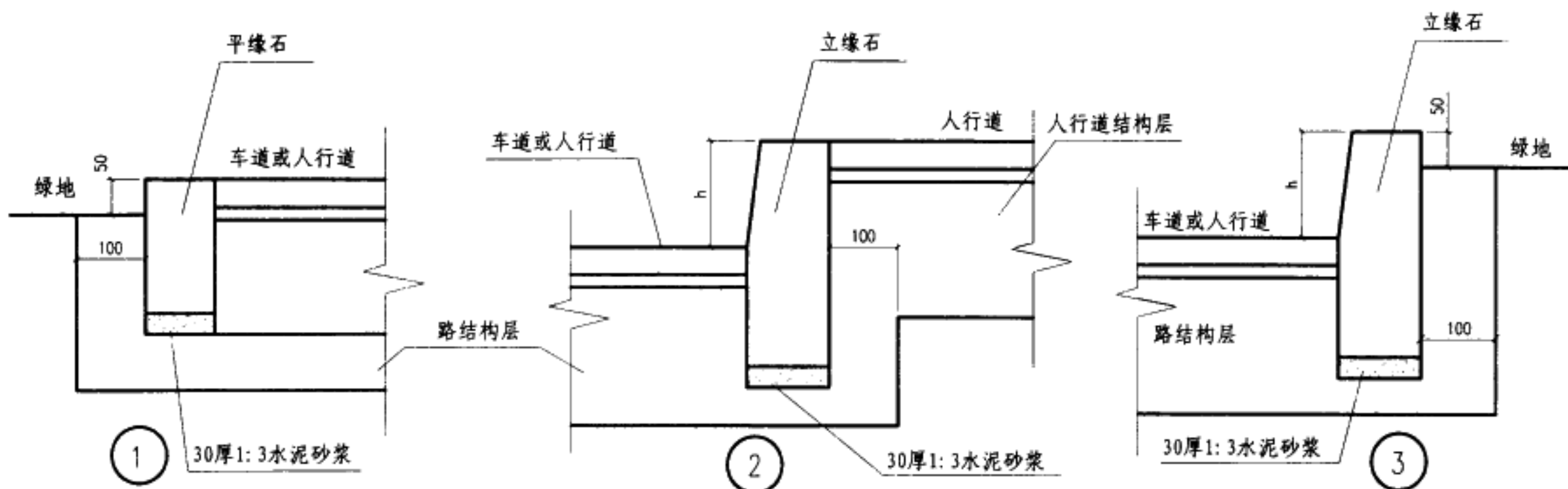
缘石安装模式
