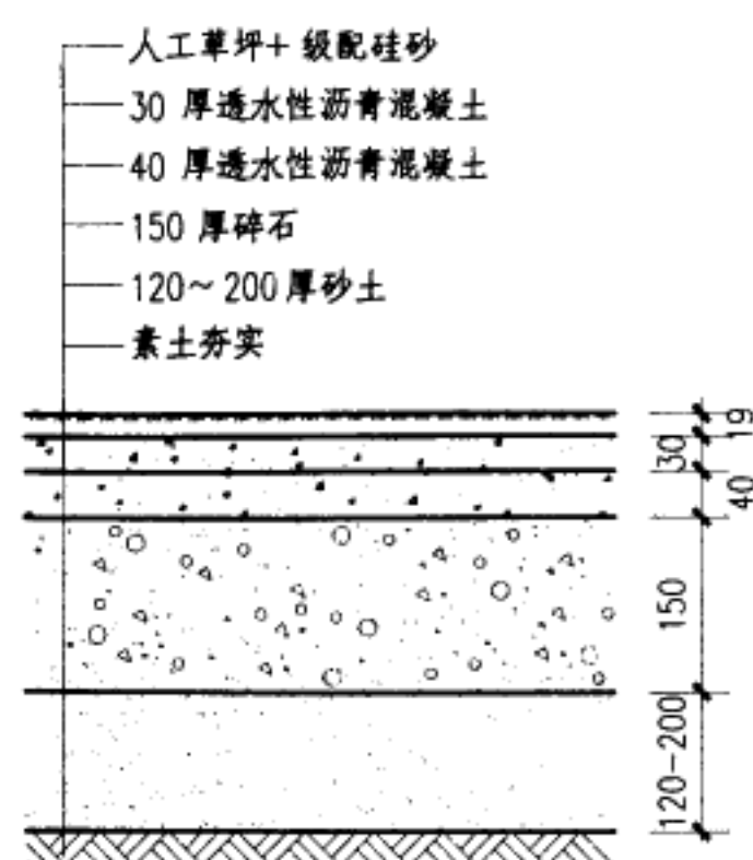
3 铺砂型人工草坪场地 (透水型)
