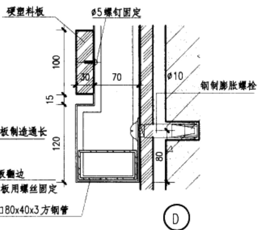
平挂式标志牌(二)
