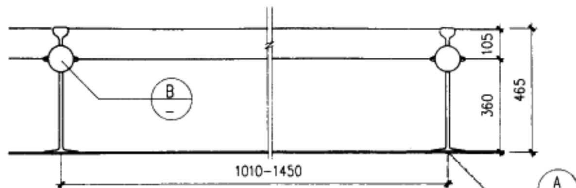
立面
