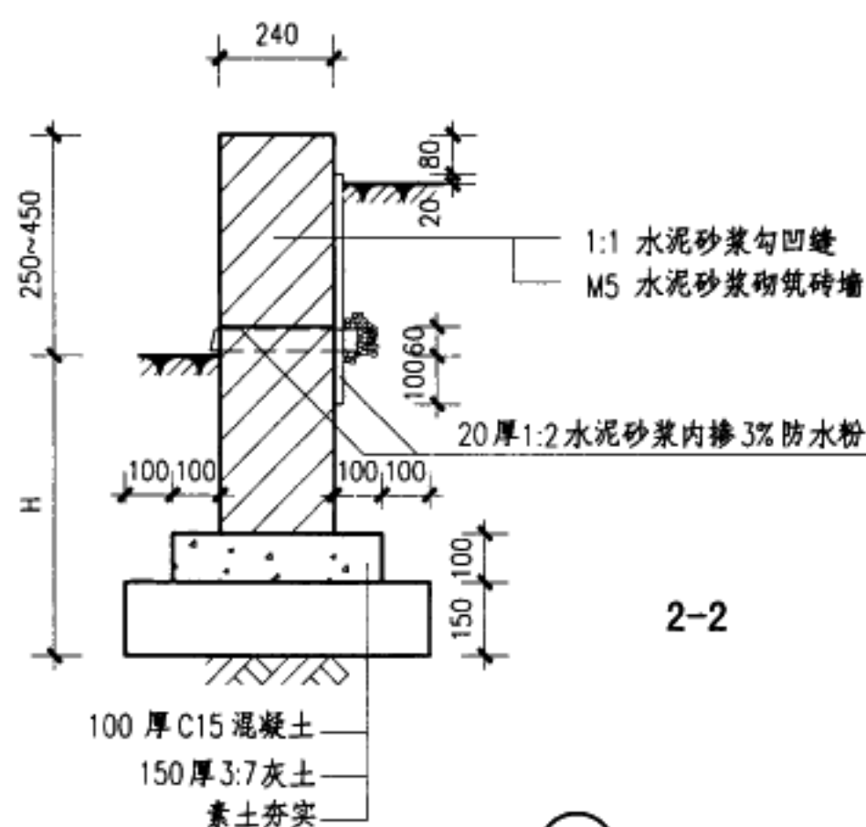
② 清水砖砌花池
