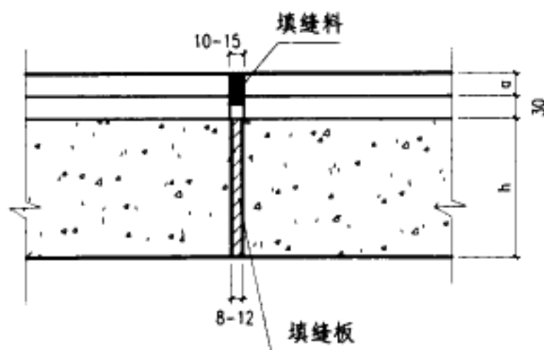
③ 上有面层, 基层为混凝土的胀缝
