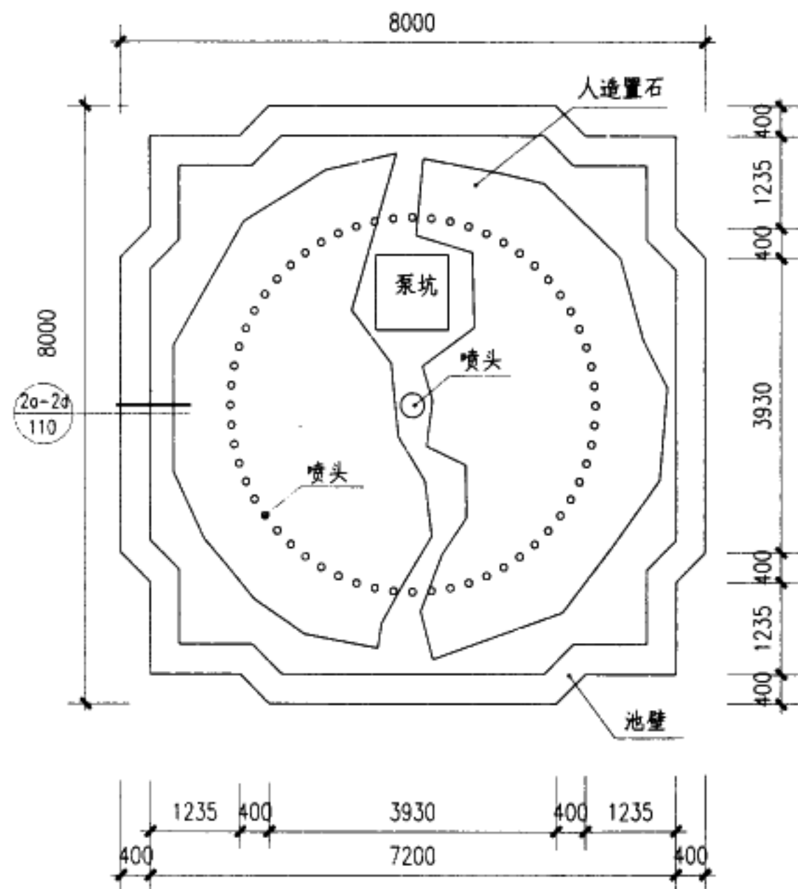
示例(二)平面
