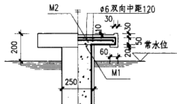
立面 剖面
