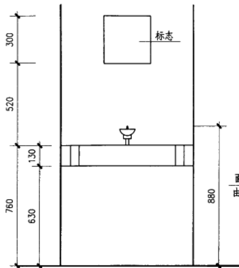
立面
