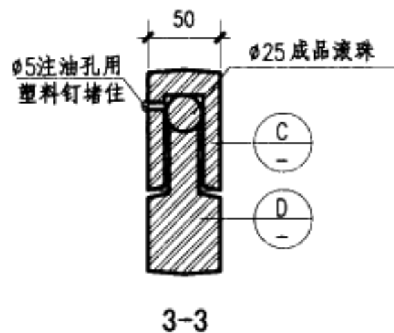
用于钢管边框门
