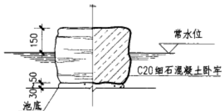
立面 剖面
