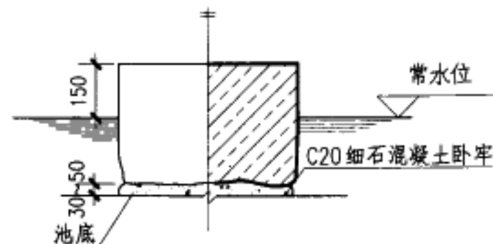
立面 剖面
