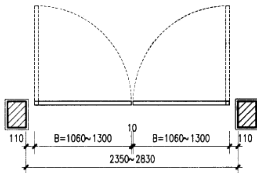
平面
