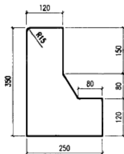
⑧ 混凝土立缘石 (120X350X745)
