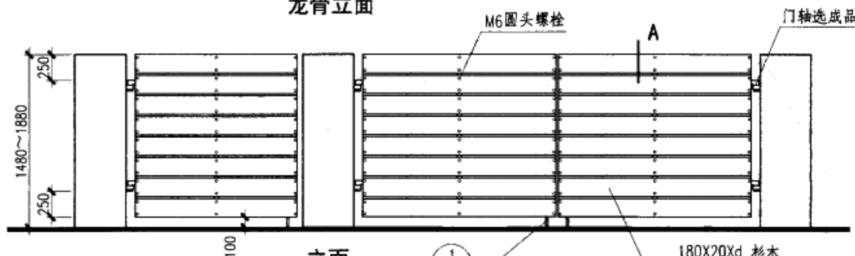
立面
