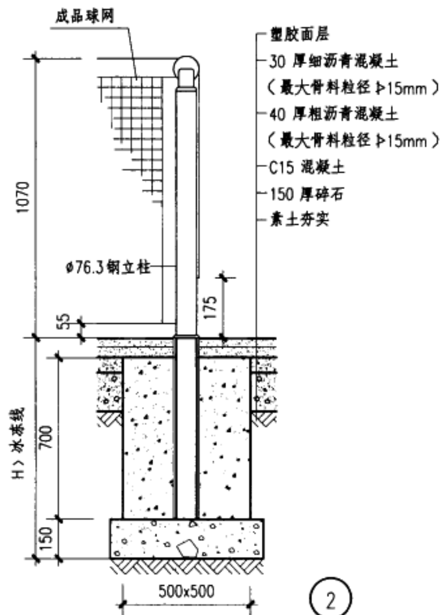
网球场组装式网柱构造详图
