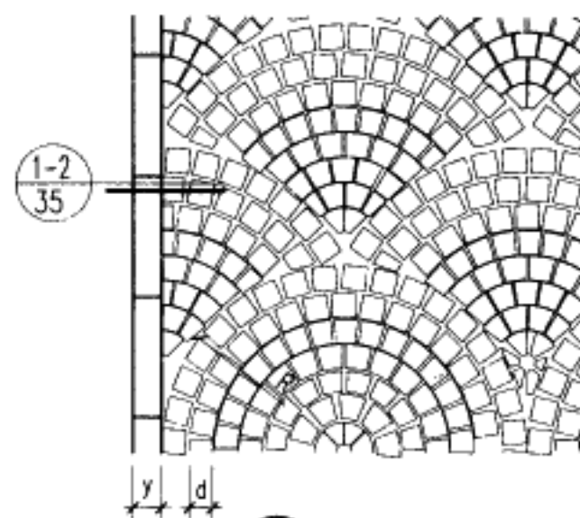
③ 花砖 小料石
