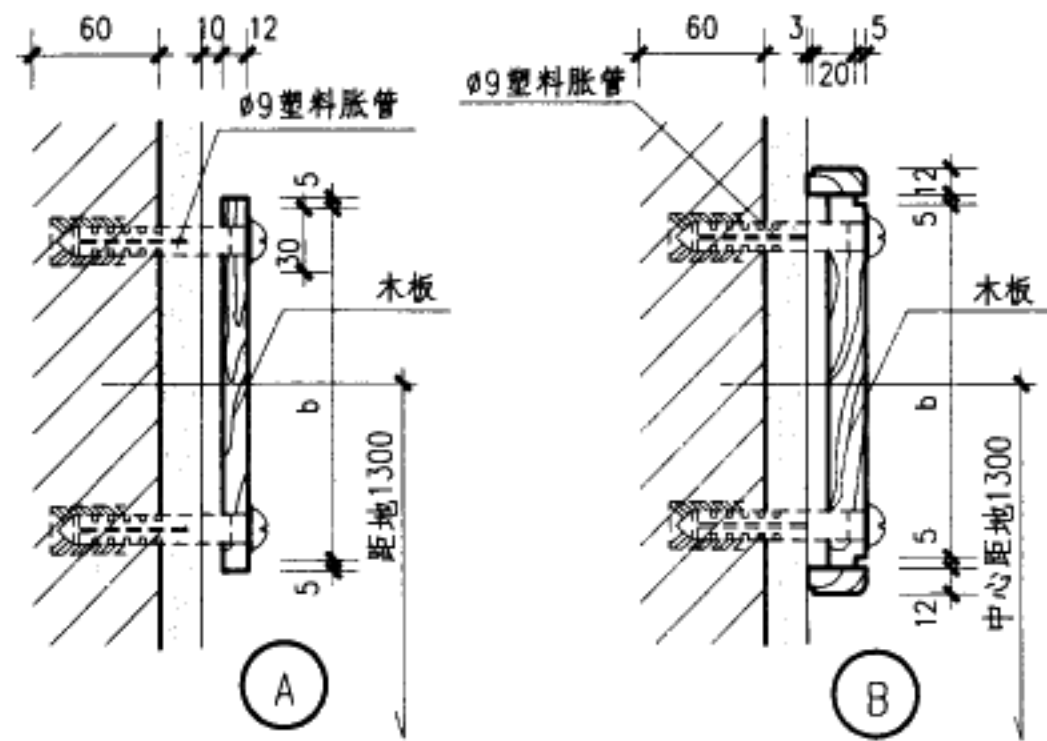
立面 ① 无框式
