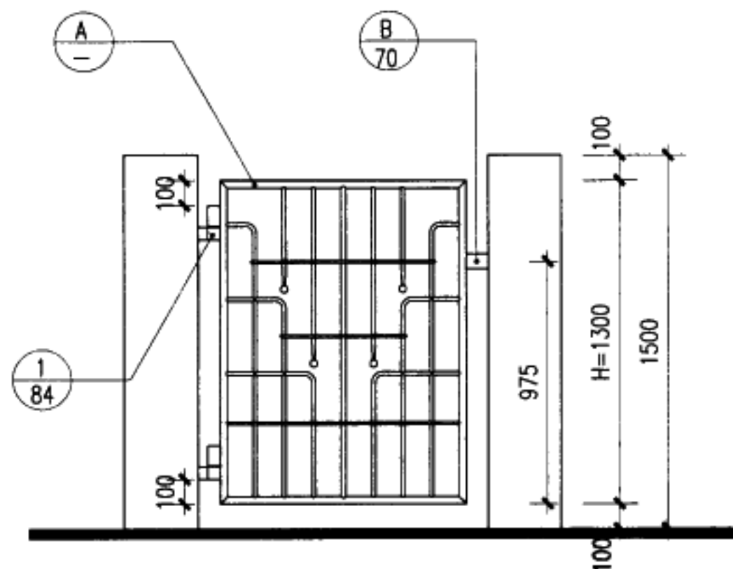
立面图
