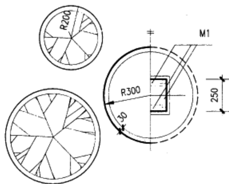
平面
