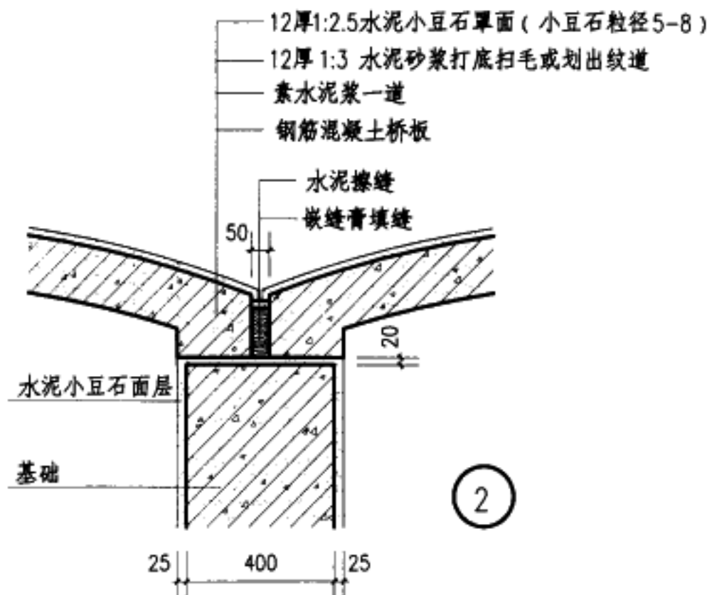
拱桥(一)
