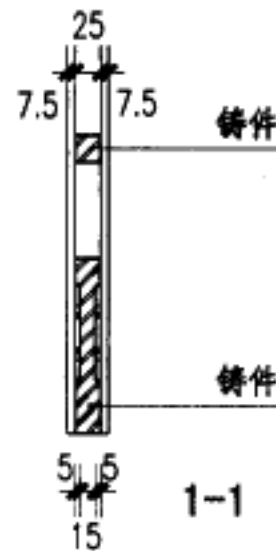
金属大门(三)
