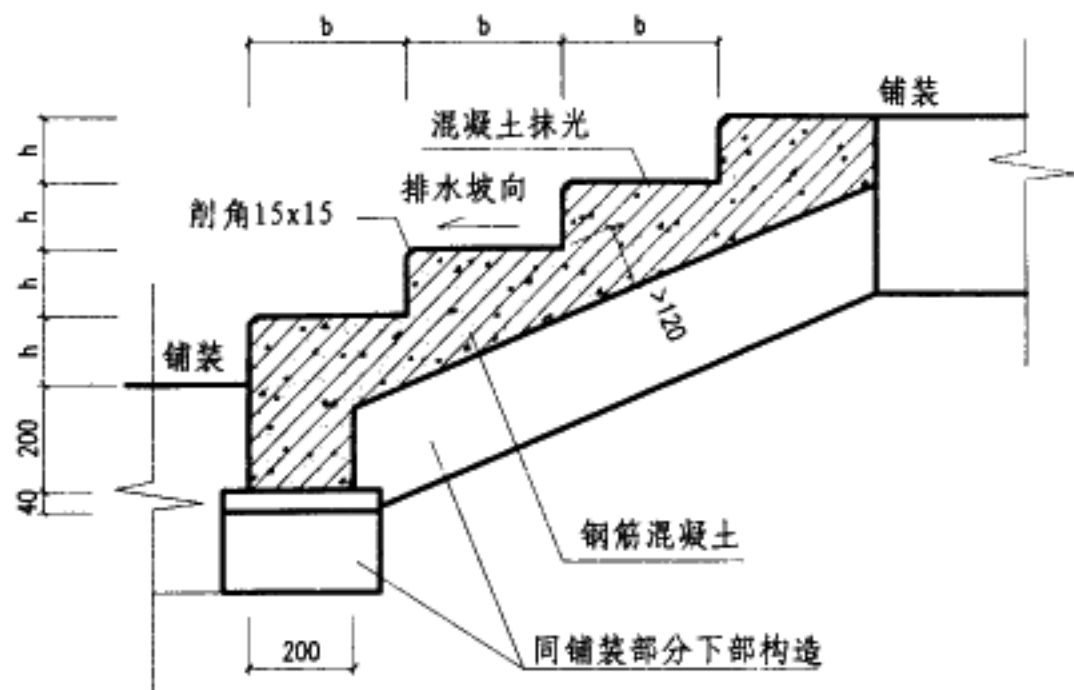
① 混凝土台阶
