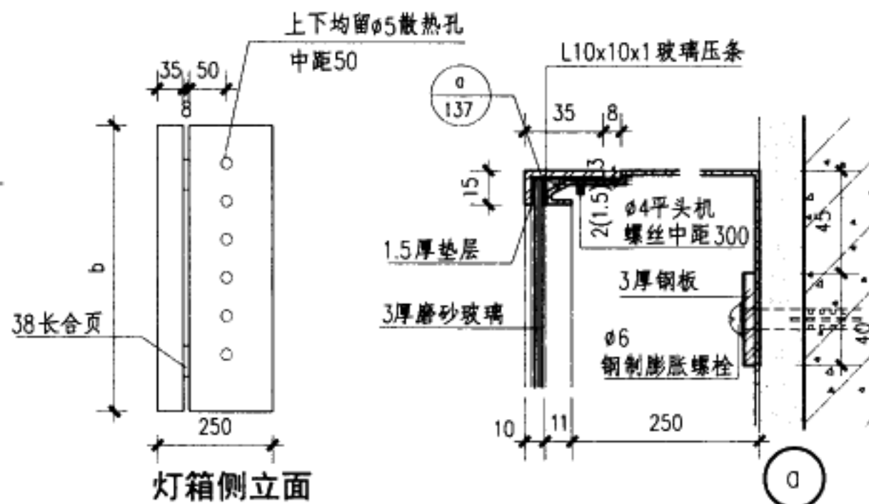
立面 ③ 灯箱式
