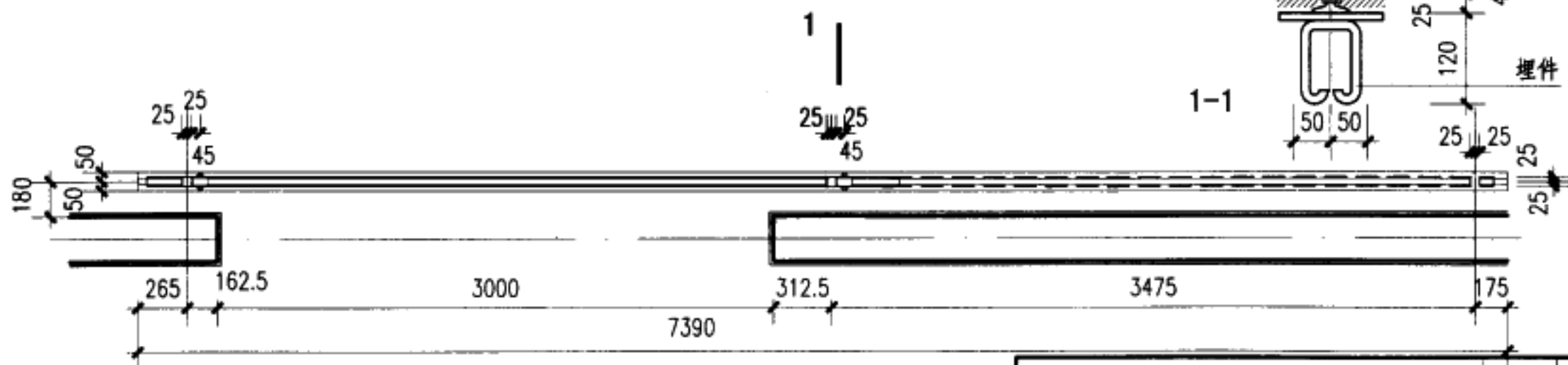
平面
