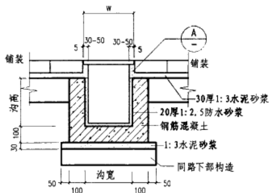
4 现场浇筑U形边沟
