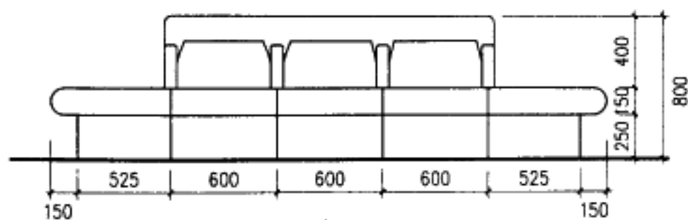
立面
