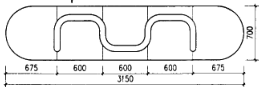
平面
