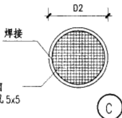
水池溢水口、排水坑、进水口 图集号 03J012-1
