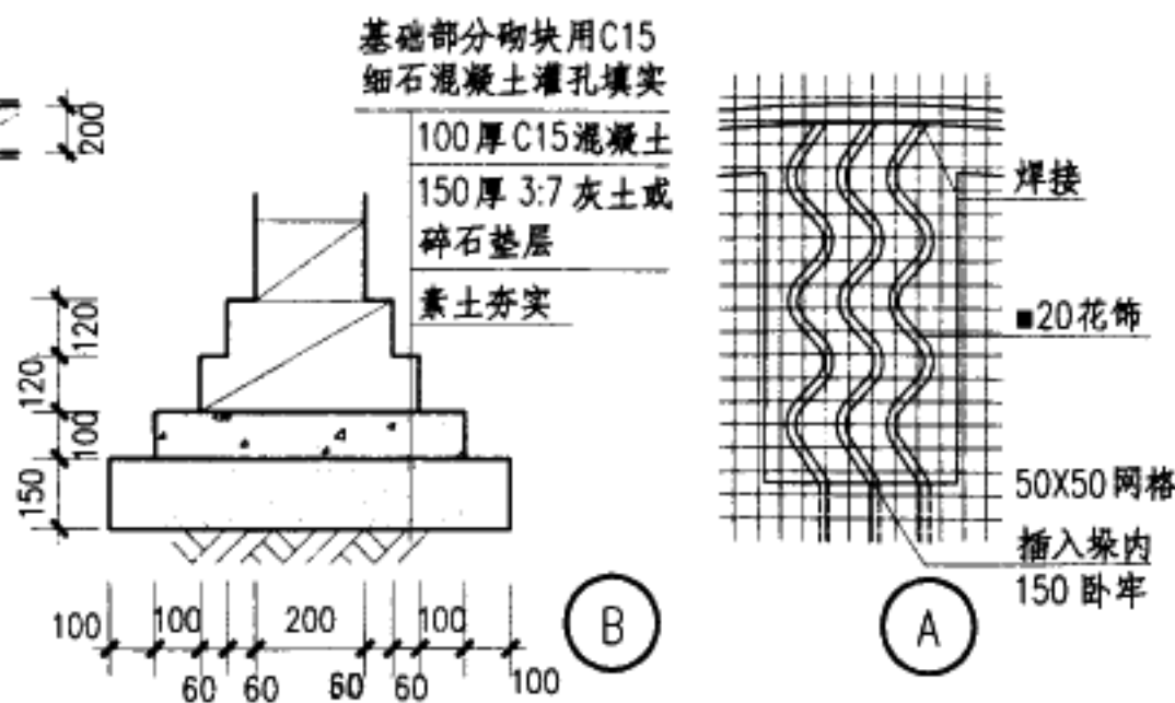
砌块铁栅围墙(二)
