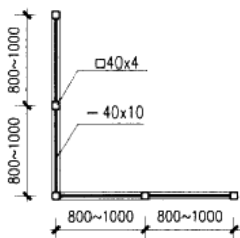
转角平面
