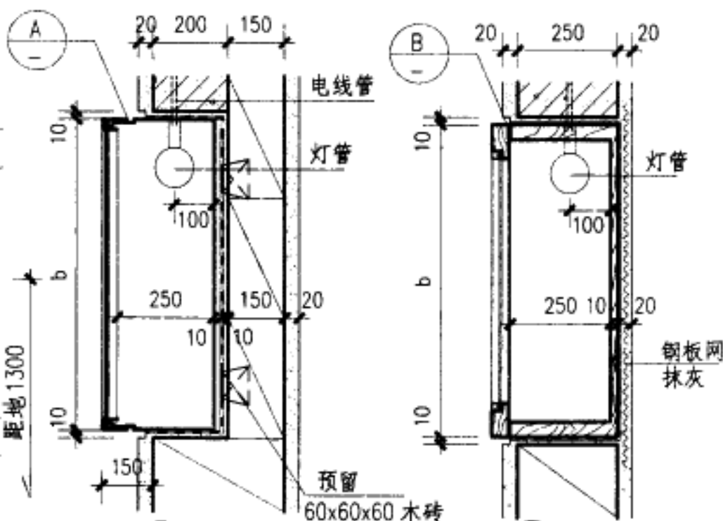
① 平挂半嵌墙式
