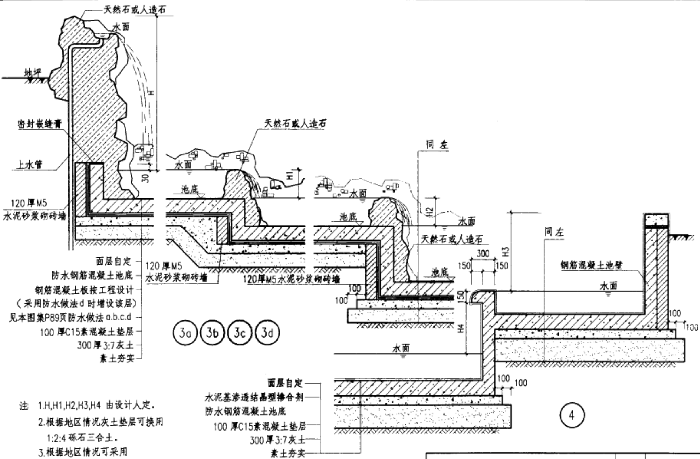
跌水 (三)
