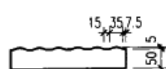
剖面
