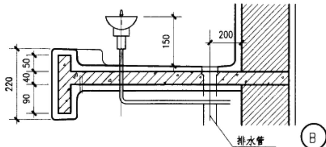
饮水台(二)
