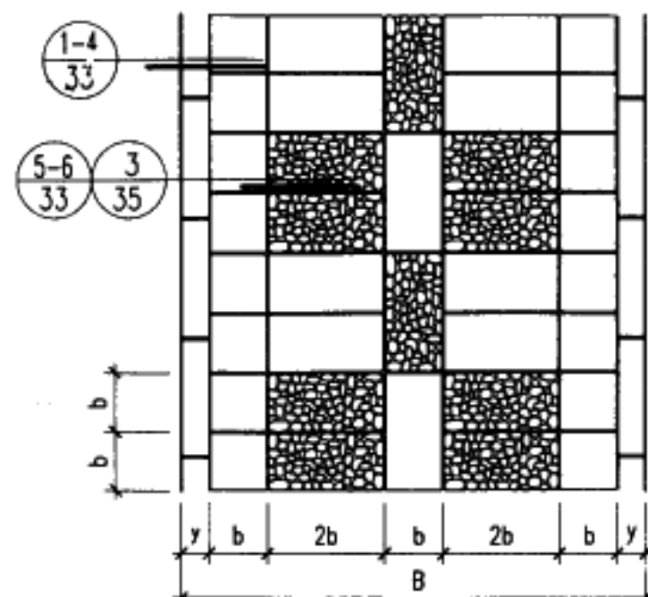
③ 水泥砖(石板)间嵌卵石(碎石)
