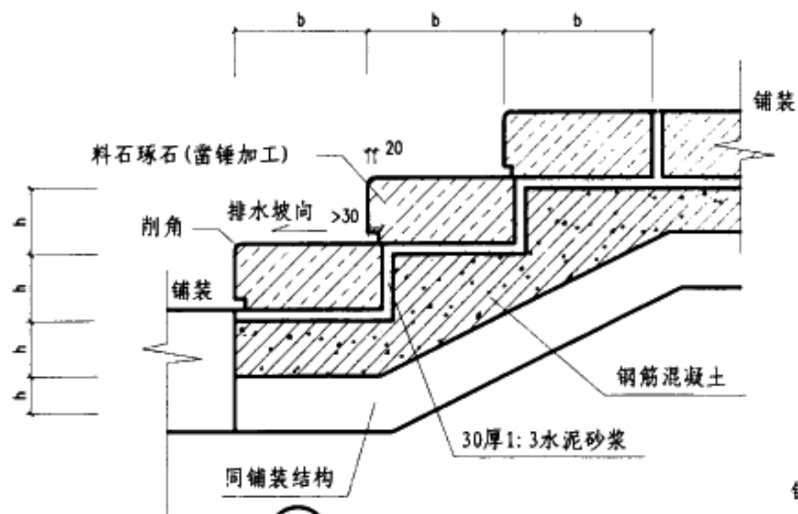
① 料石台阶
