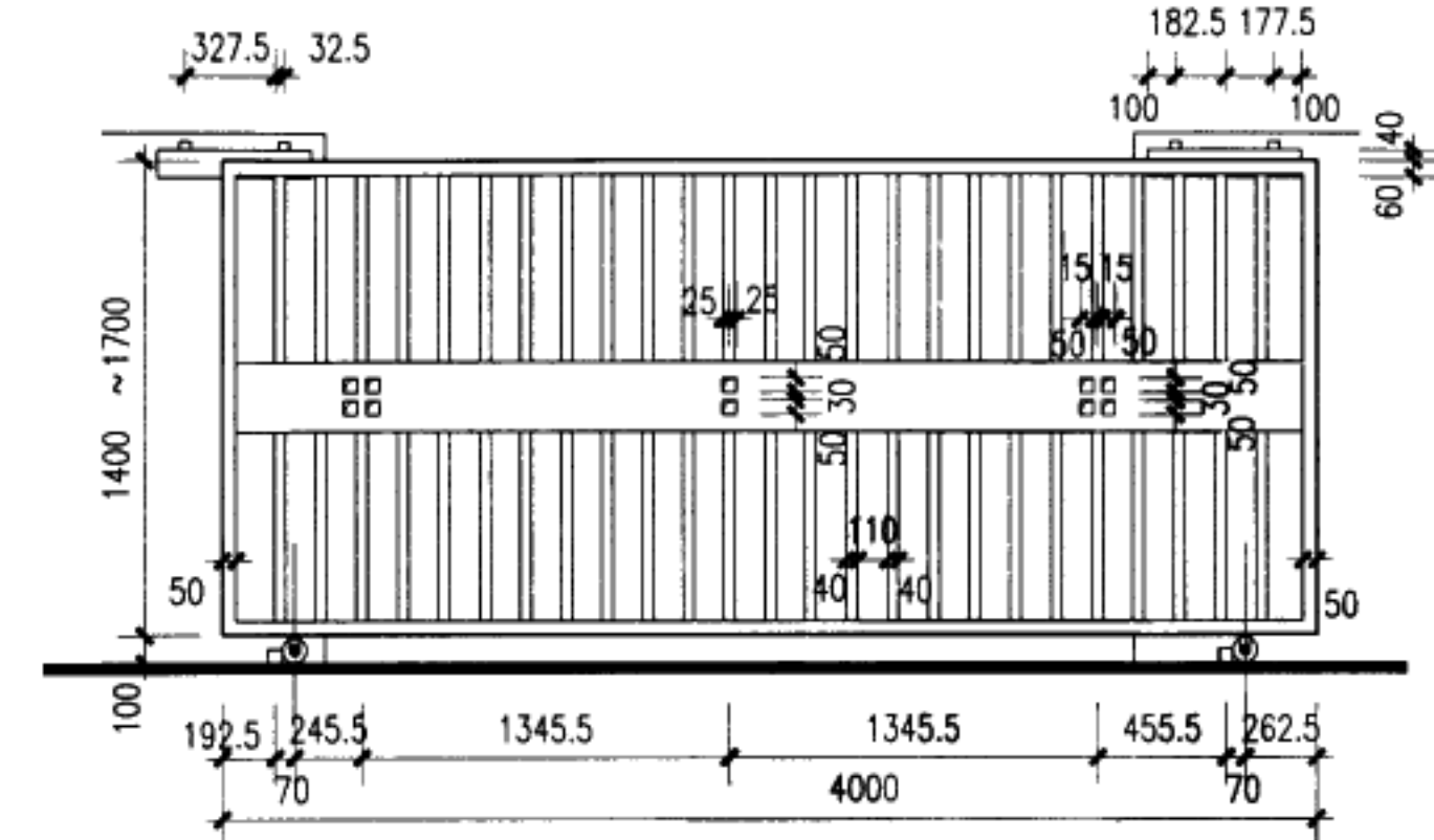
立面
