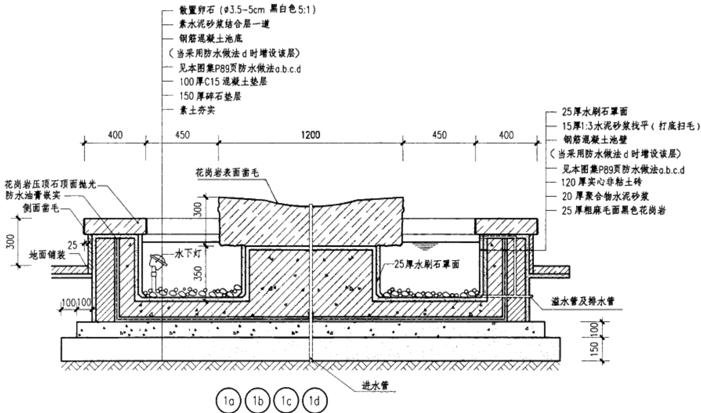
喷泉示例(一)剖面图
