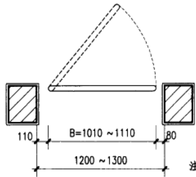
平面图
