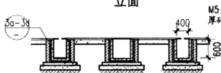
立面
