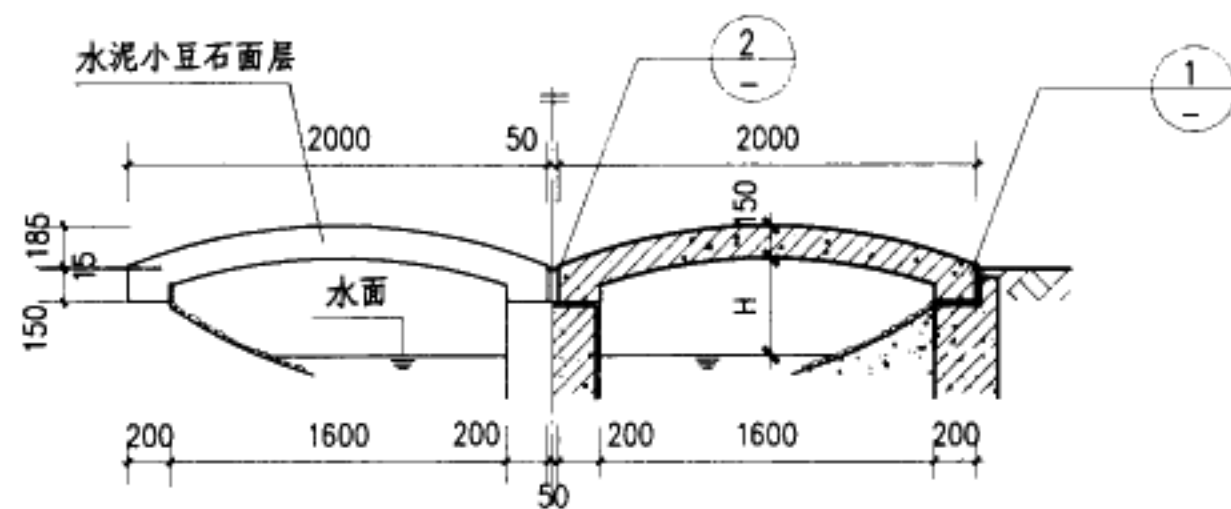
立面
