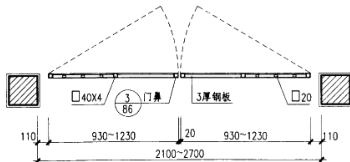
平面
