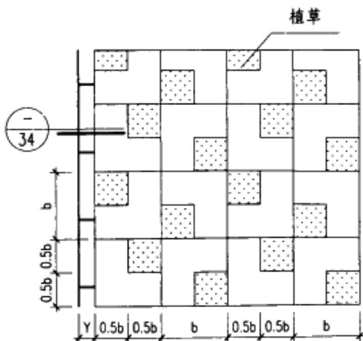
④ 型嵌草砖
