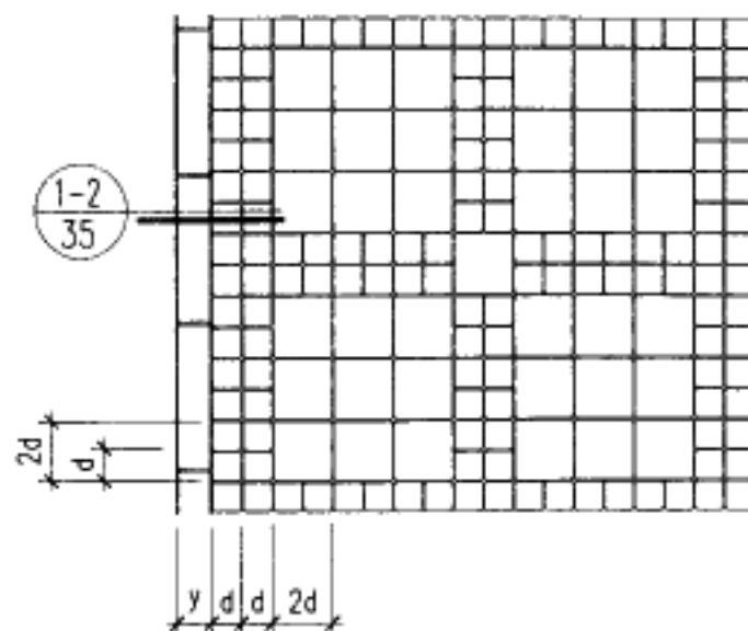
④ 花砖 小料石
