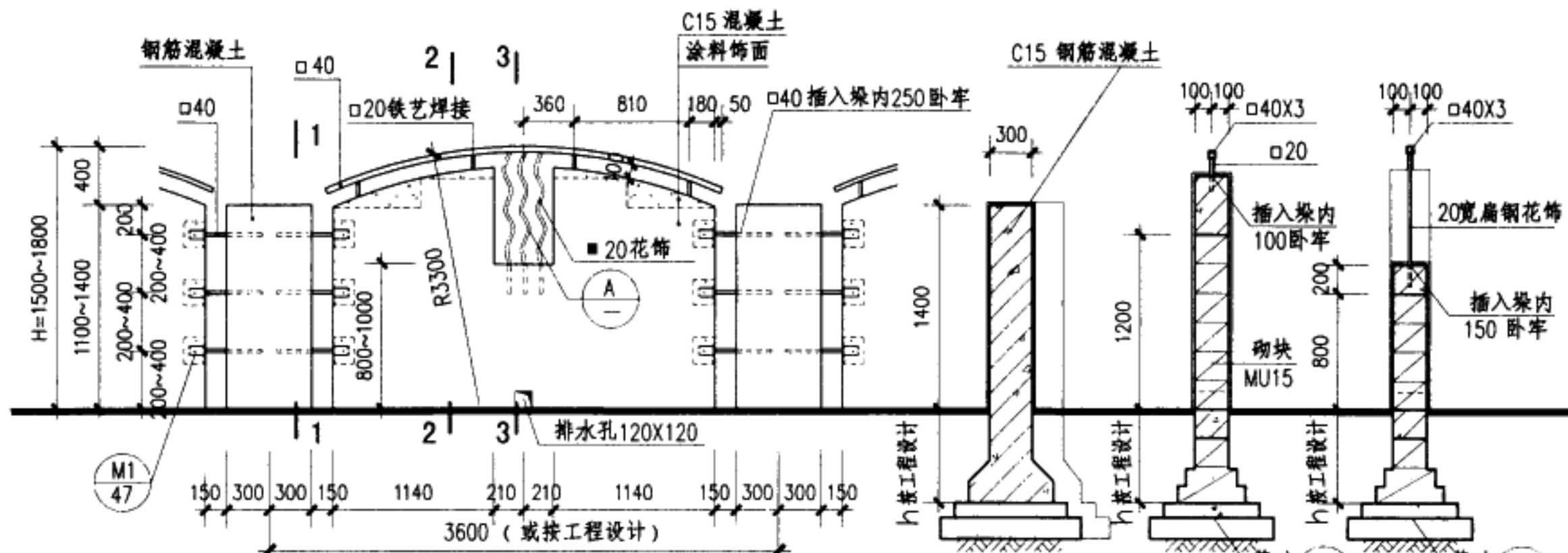
立面
