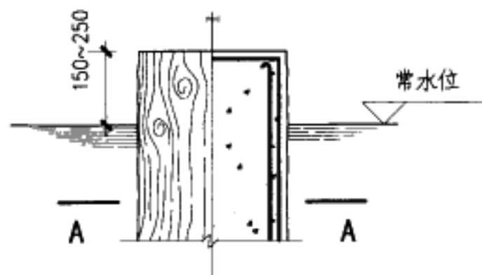
立面 剖面
