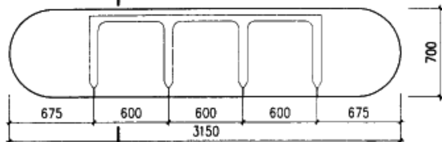
平面
