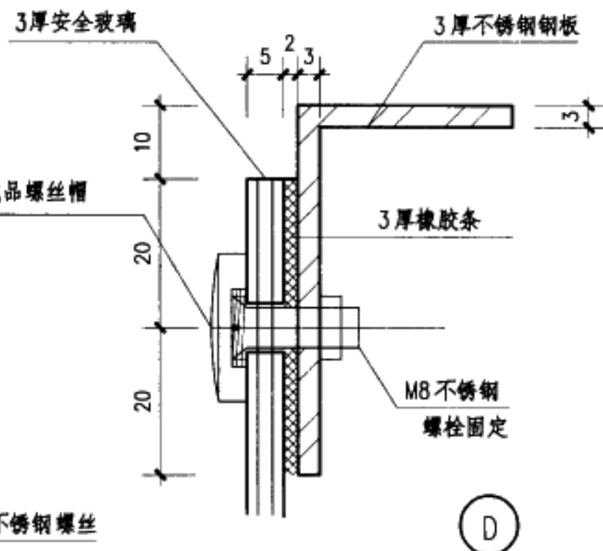
吊挂节点详图(一)
