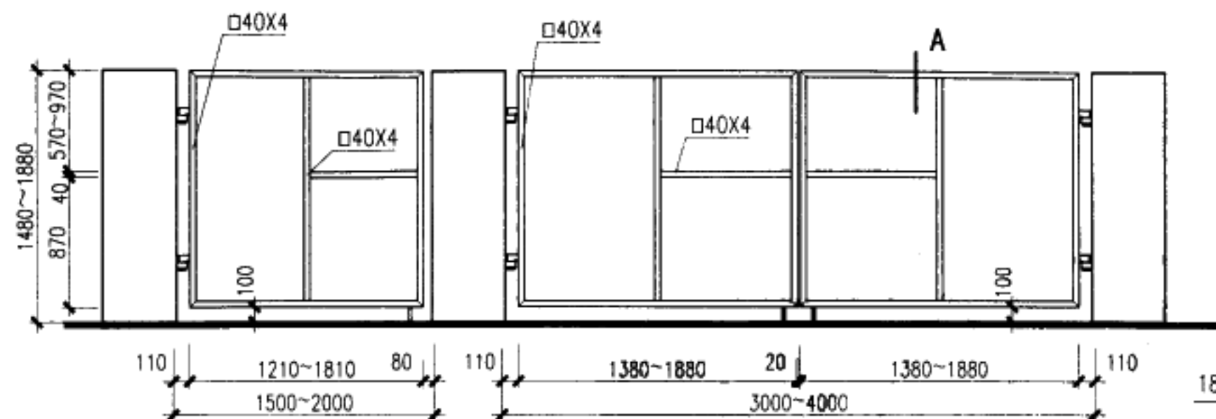
龙骨立面
