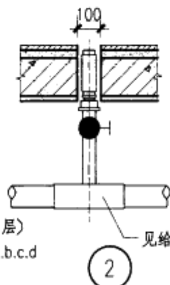
旱喷示例(二)
