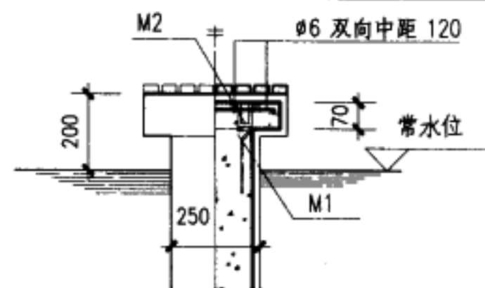
立面 剖面
