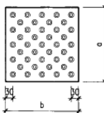
平面
