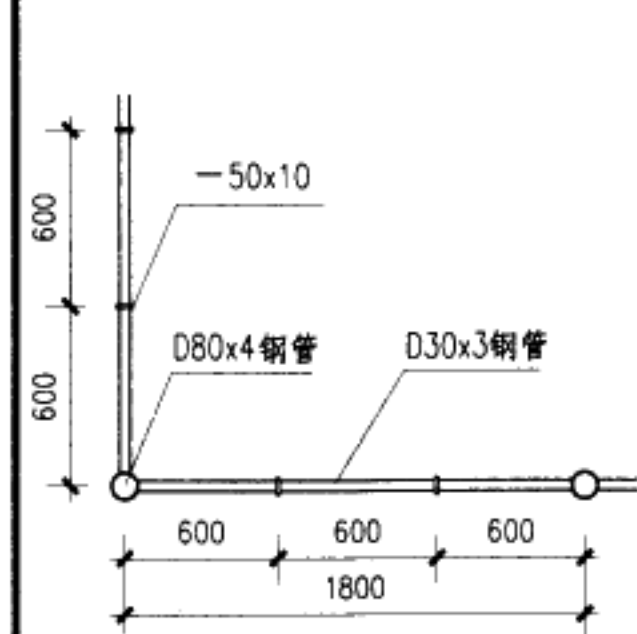
转角平面
