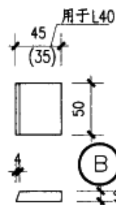
门轴详图 (三)
