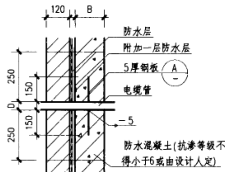
3 电缆管道穿池壁
