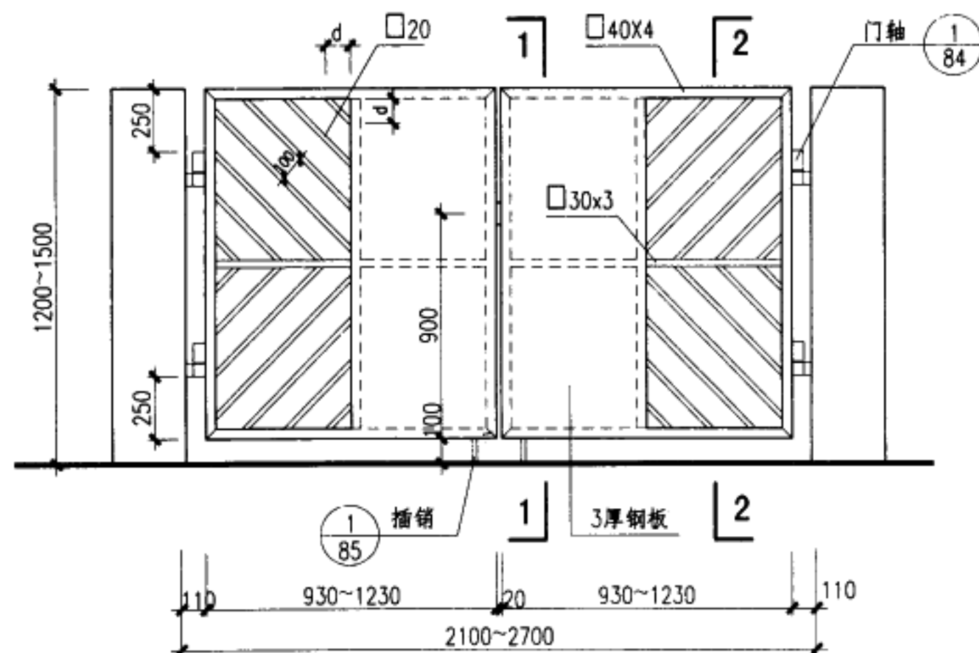
立面
