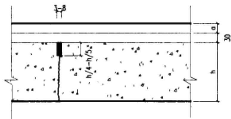
④ 上有面层, 基层为混凝土假缝
