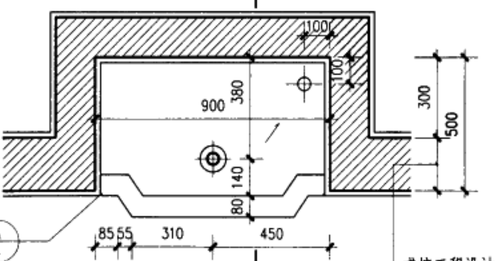
平面
