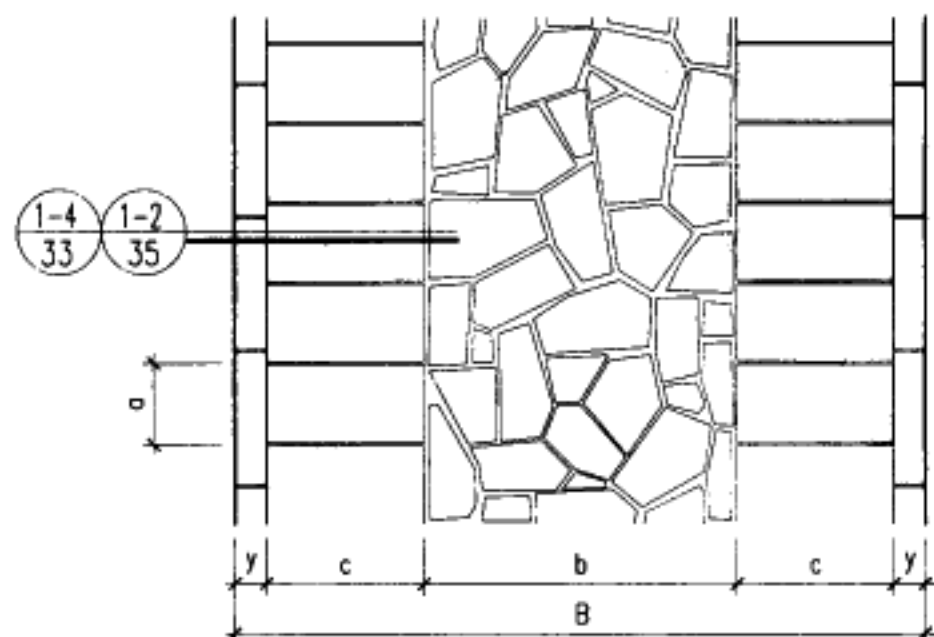
④ 碎石板与水泥砖(石板)组合
