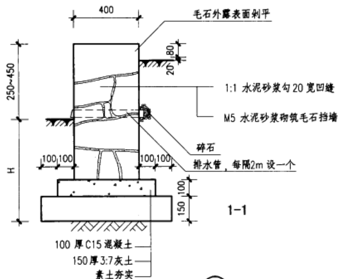
① 毛石花池
