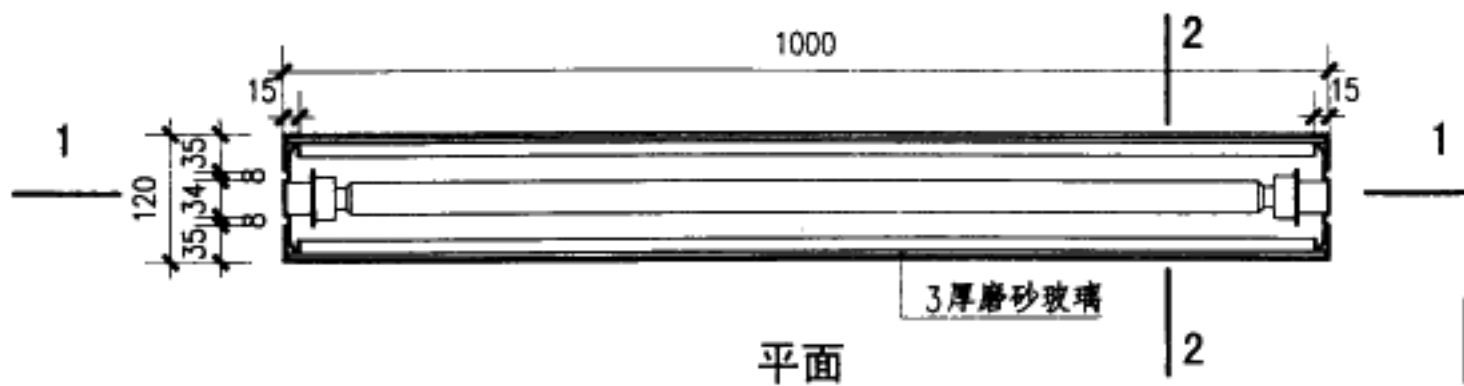
顶挂式(照明)标志牌(二)
