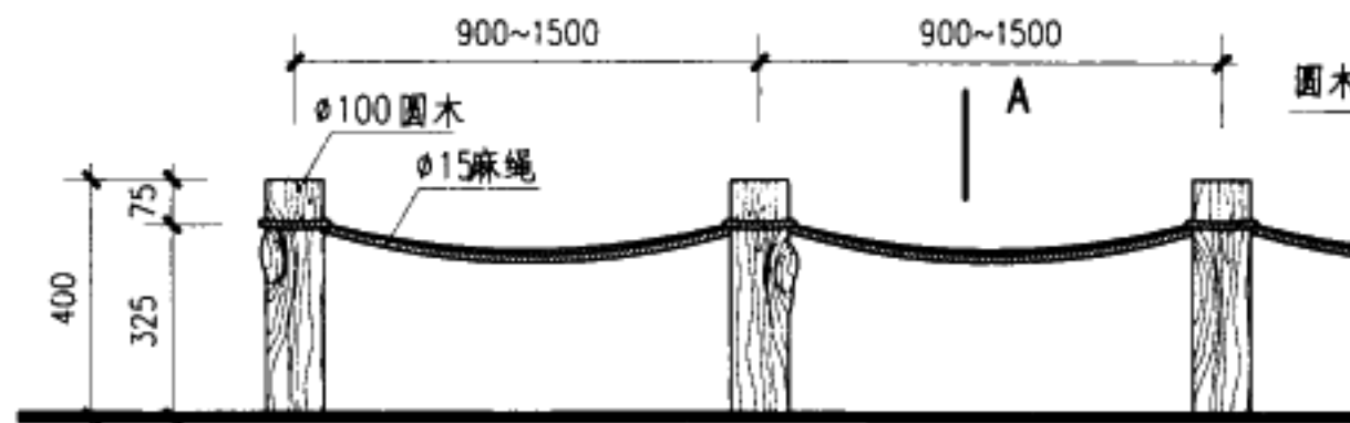
立面
