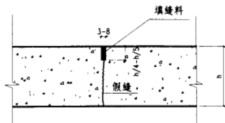
① 假缝型缩(纵)缝
