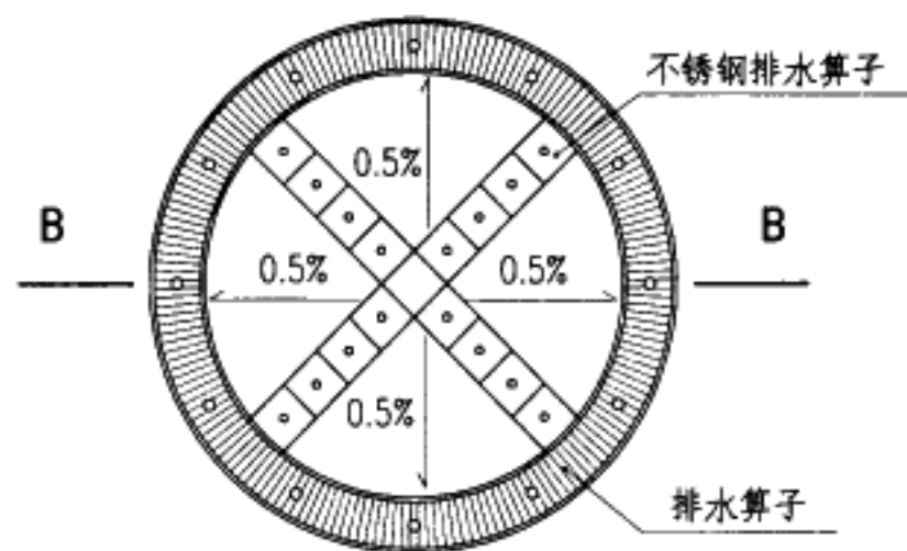
平面
