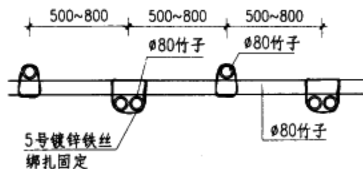
平面
