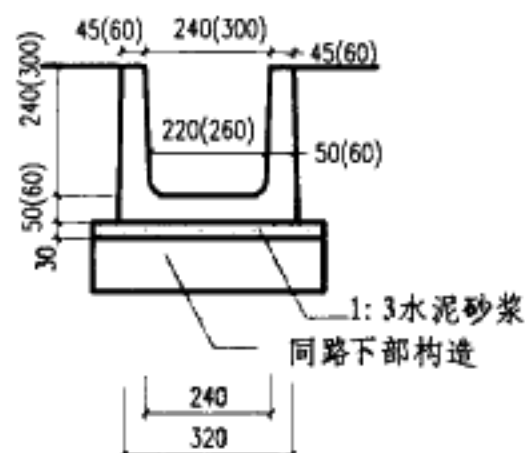
2 预制U形边沟
