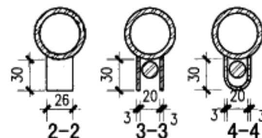
门轴详图(六)
