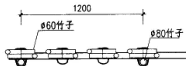
平面
