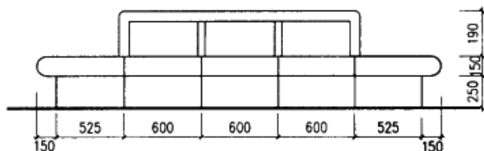
立面
