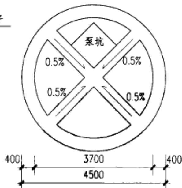
坑底平面
