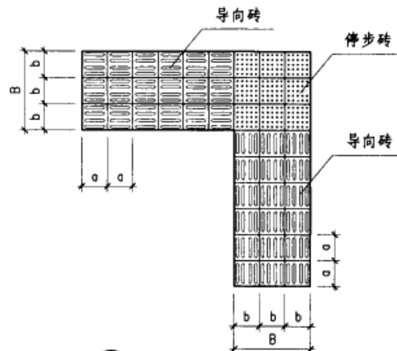
③ 盲道砖铺装样式
