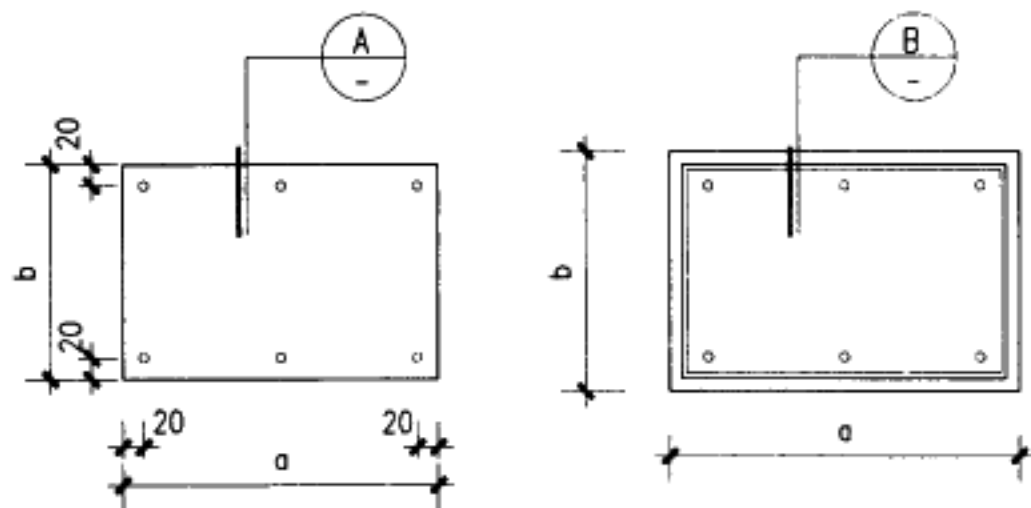
立面 ① 无框式
