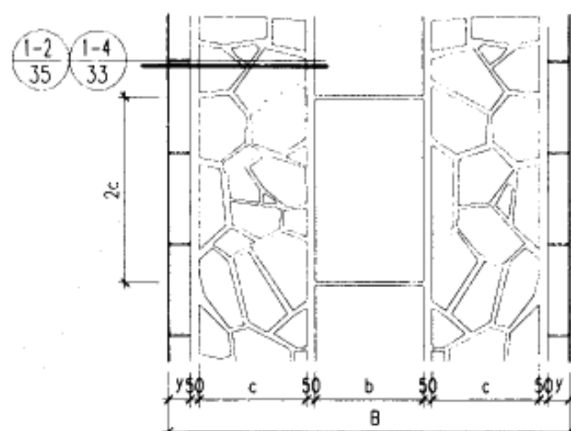
③ 碎石板与水泥砖(石板)组合
