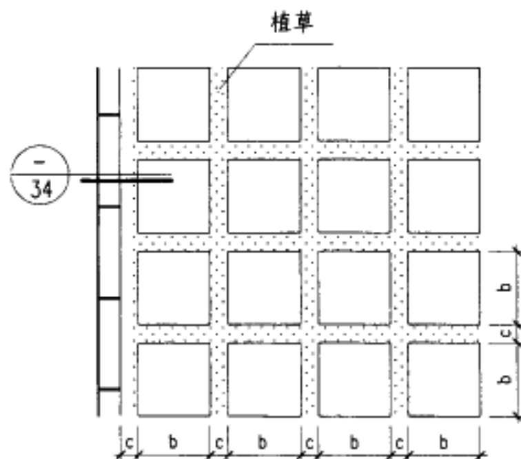
⑤ 水泥砖间嵌草
