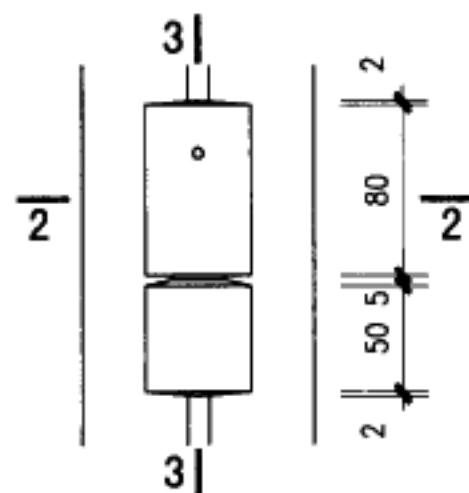
② 相联门轴 (用于四扇门)
