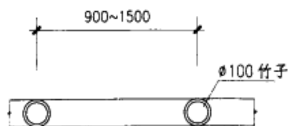
平面
