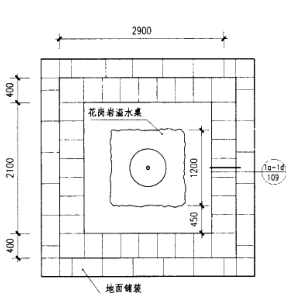
示例(一)平面
