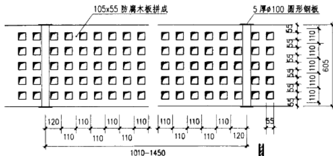
平面
