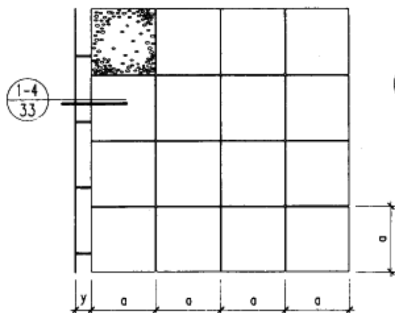
④ 预制嵌卵石水泥砖
