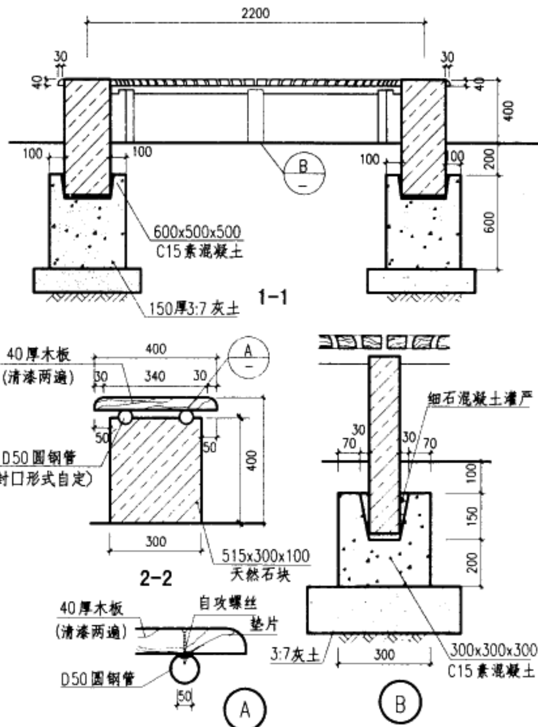
木制围树椅(二)
