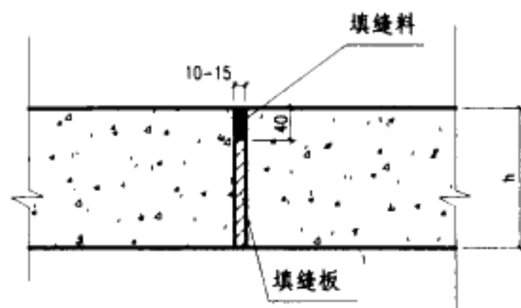
② 混凝土路的胀缝
