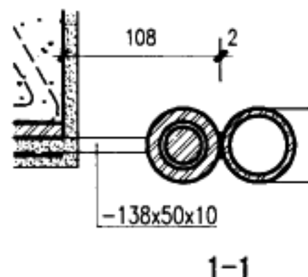
用于钢管边框门
